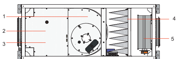
Rys. 4.6.1. AmberAir Compact VEKA INT EKO 400/700
