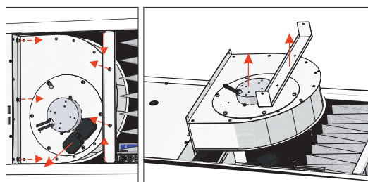
Rys. 6.5.1. AmberAir Compact VEKA INT 400-700 EKO
