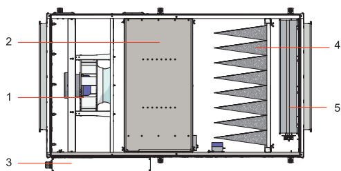
Rys. 4.6.3. AmberAir Compact VEKA INT EKO 3000/4000
