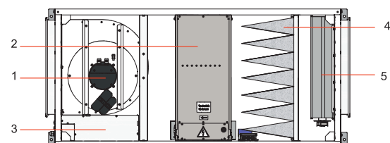
Rys. 4.6.2. AmberAir Compact VEKA INT EKO 1000/2000
