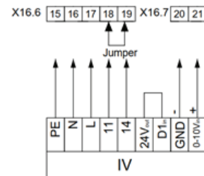
Extract air fan (max. 6A)
