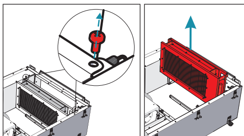
Rys. 6.6.3. AmberAir Compact VEKA INT W EKO
