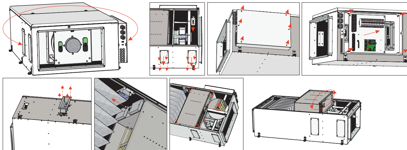
Rys. 5.5.3. AmberAir Compact VEKA INT 1000-4000 EKO zmiana strony obsługowej
