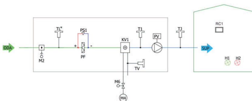
Rys. 5.4.1. AmberAir Compact VEKA INT W EKO (* W centralach AmberAir Compact VEKA 1000-2000 TL znajduje się na zewnątrz urządzenia, po lewej stronie M2)
