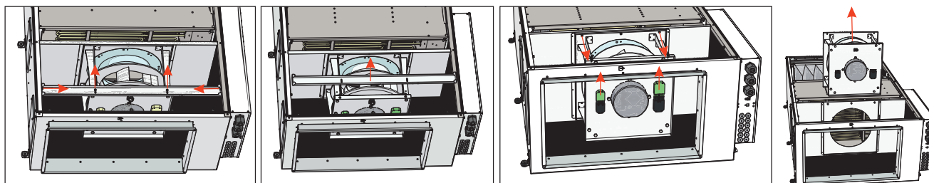
Rys. 6.5.2. AmberAir Compact VEKA INT 1000-4000 EKO
