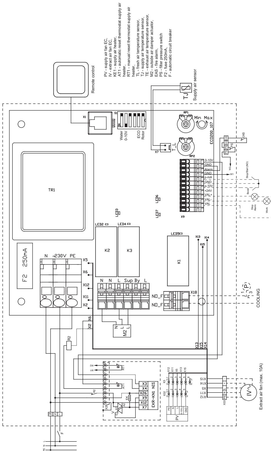
Rys. 8.7.1. AmberAir Compact VEKA INT EKO 400-1.2; 2.0; 700-2.4
