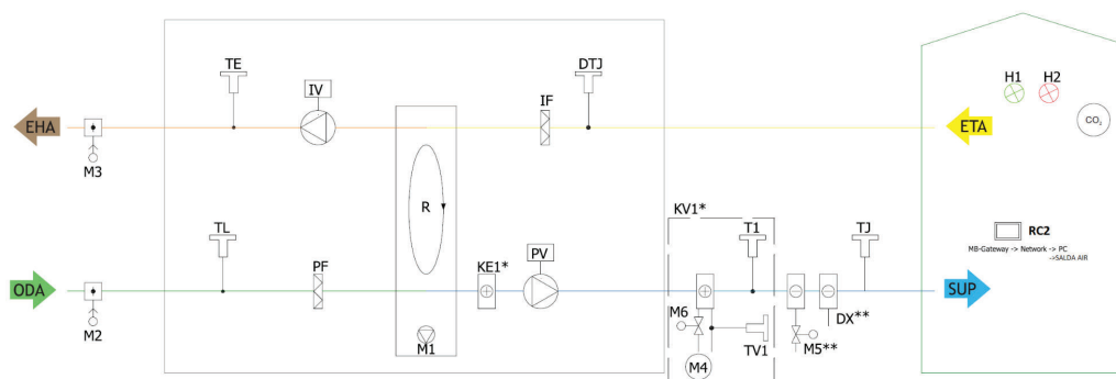
Рисунок 5.4.1. * KE1 - только в электрическом исполнении; * KV1 - используется в водном исполнении; ** Возможно управление.
