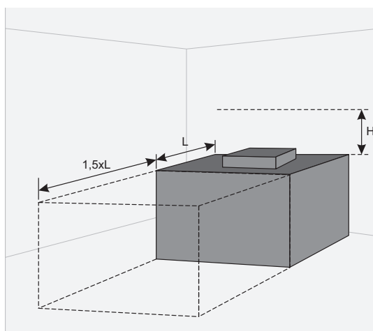
Рисунок 5.5.1.1. Мин. расстояние до открытия двери - 1,5 \times L ; Мин. расстояние до открытия двери блока управления - H > 400 мм.
