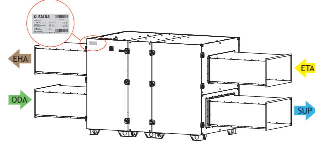
Pav. 3.3.6 Techninio lipduko vieta ir oro kanalų žymėjimas AmberAir Compact-S-R-3000-H (dešininė versija)
