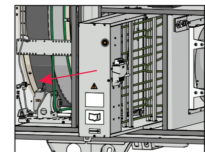
Pav. 6.8.2 Šildytuvo išėmimas
