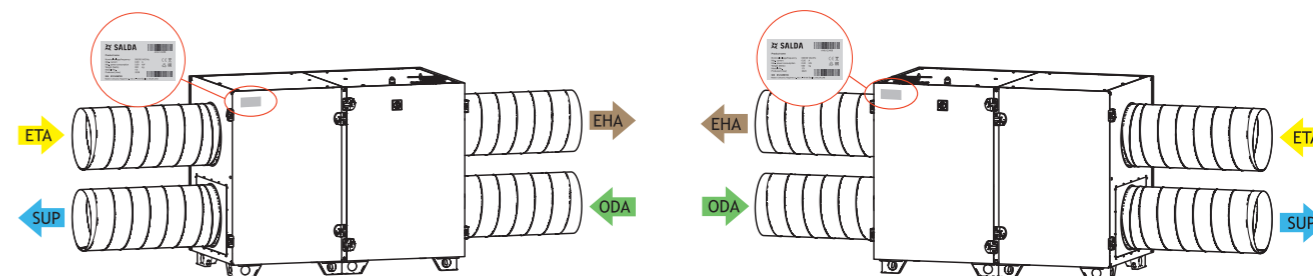
Pav. 3.3.3 Techninio lipduko vieta ir oro kanalų žymėjimas AmberAir Compact-S-R-1000-2000-H (kairinė versija)
