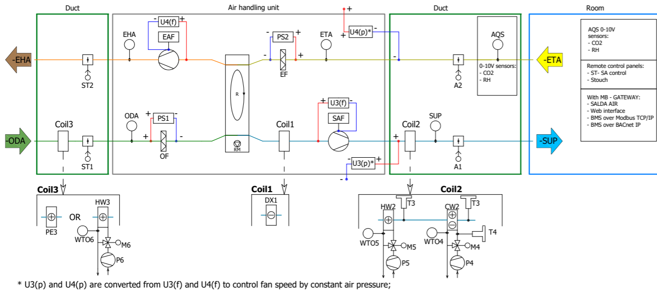
Pav. 8.6.3 Horizontalūs dešinieji įrenginiai su integruota DX aušinimo rite
