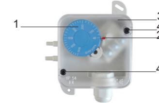
1 - skydas su slėgio vertėmis; 2 - ženklas; 3 - dangtelis; 4 - tvirtinimo varžtai.
