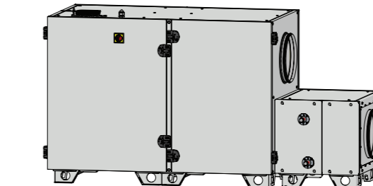
Pav. 4.10.1 Išorinio šildytuvo / aušintuvo jungtis
