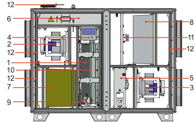
Pav. 9.2.1 AmberAir Compact S-R H
