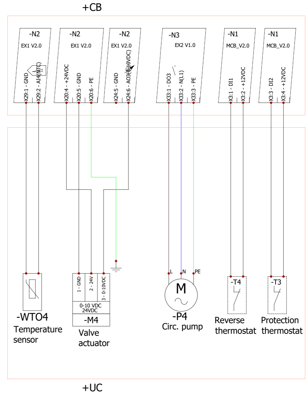
Pav. 4.18.3.2 Išorinės bendros šildymo / aušinimo ritės prijungimas
