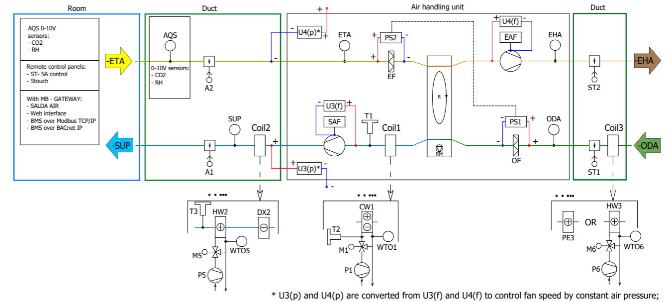
Pav. 8.6.5 Horizontalūs kairiniai įrenginiai su integruota šildymo / aušinimo rite
