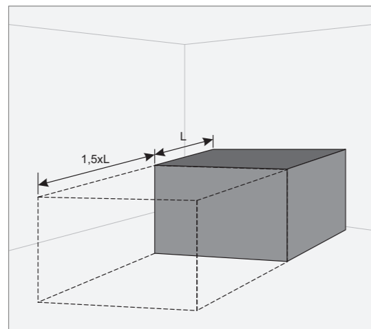
Pav. 4.7.2 Minimalus atstumas durims atidaryti - 1,5xL
