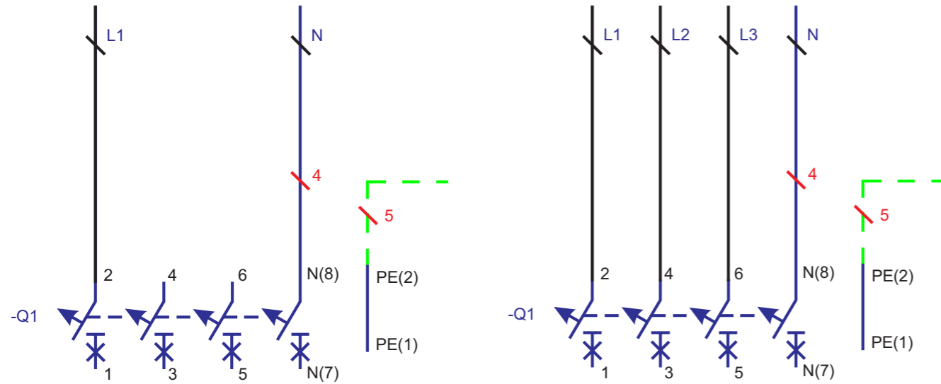
Pav. 4.15.1 Įrenginiai su 1N~ 230V maitinimo šaltiniu
