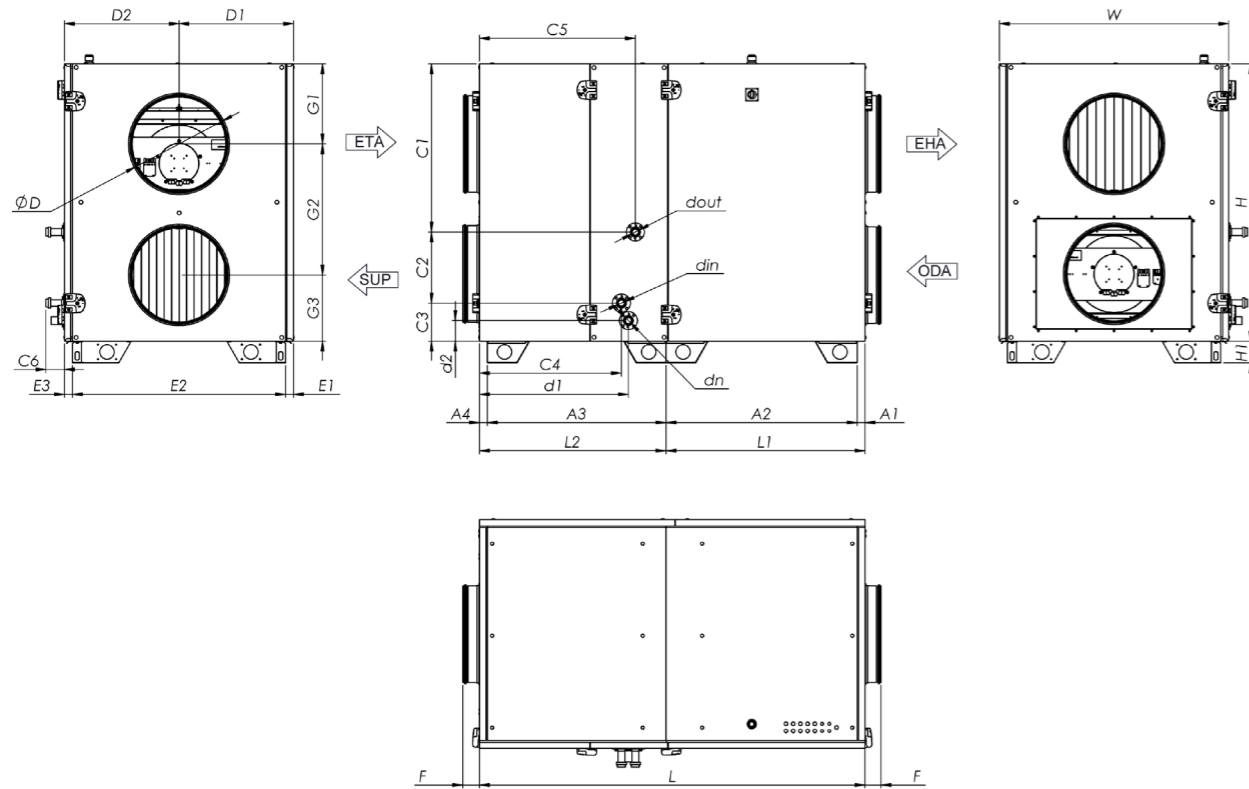
Pav. 8.1.9 AmberAir Compact-S-R-2000-H-CO-L-C1 matmenys
