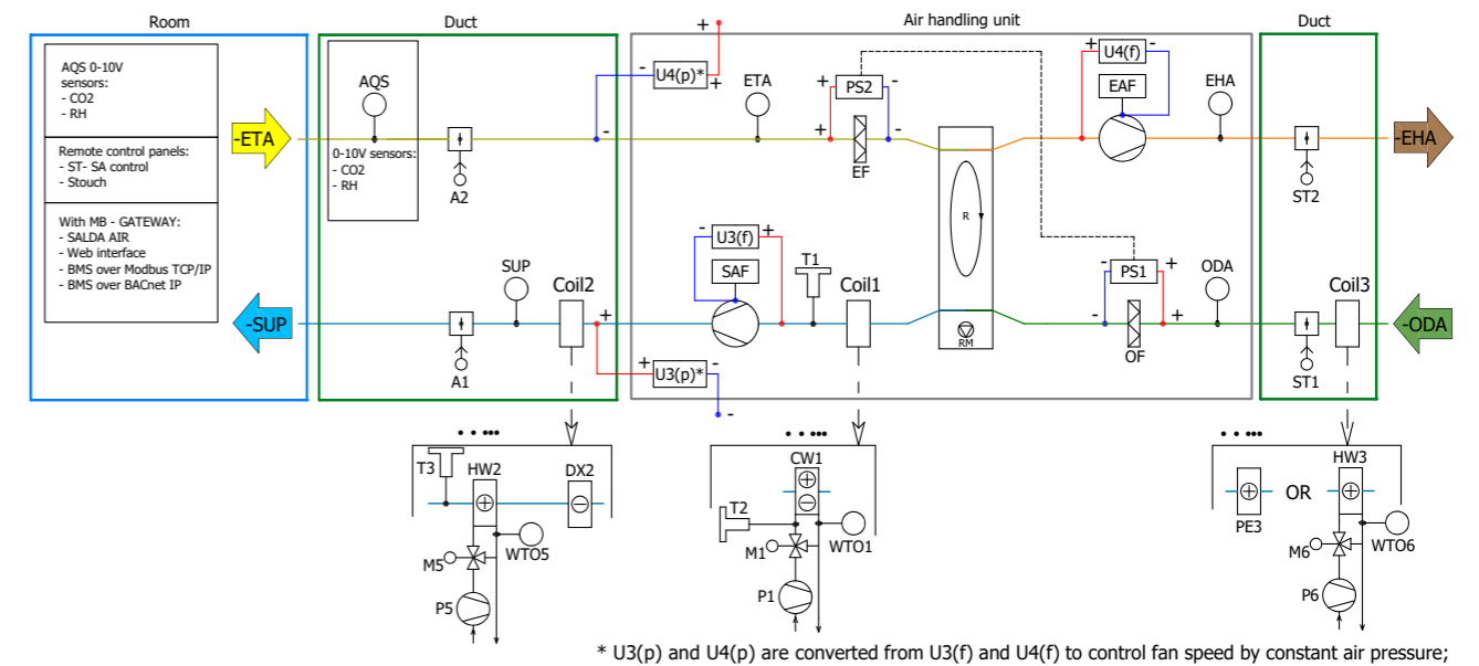
Pav. 8.6.6 Horizontalūs kairieji įrenginiai su integruota DX aušinimo rite
