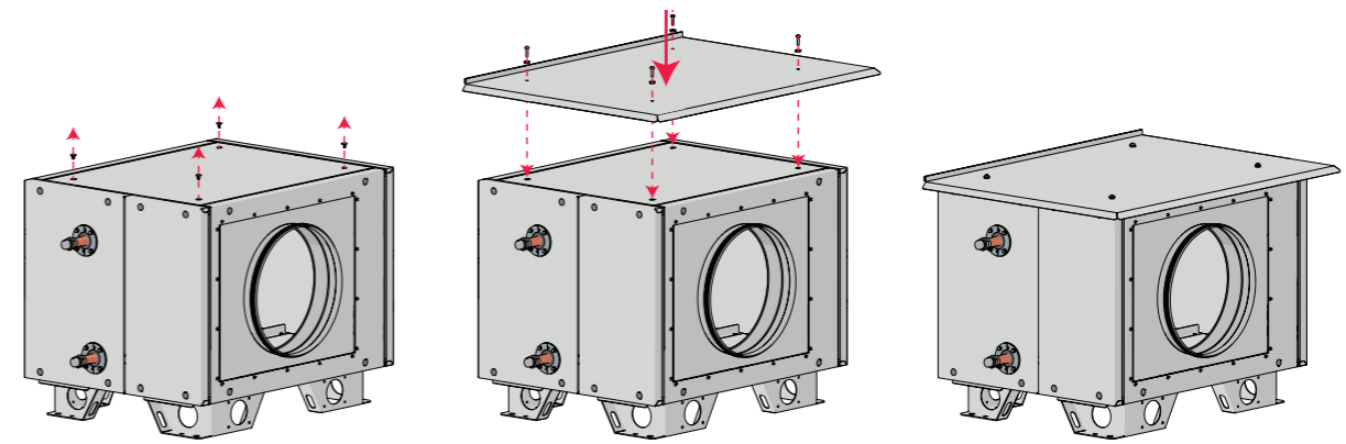
Pav. 4.10.2 Išorinio šildytuvo / aušintuvo stogo montavimas
