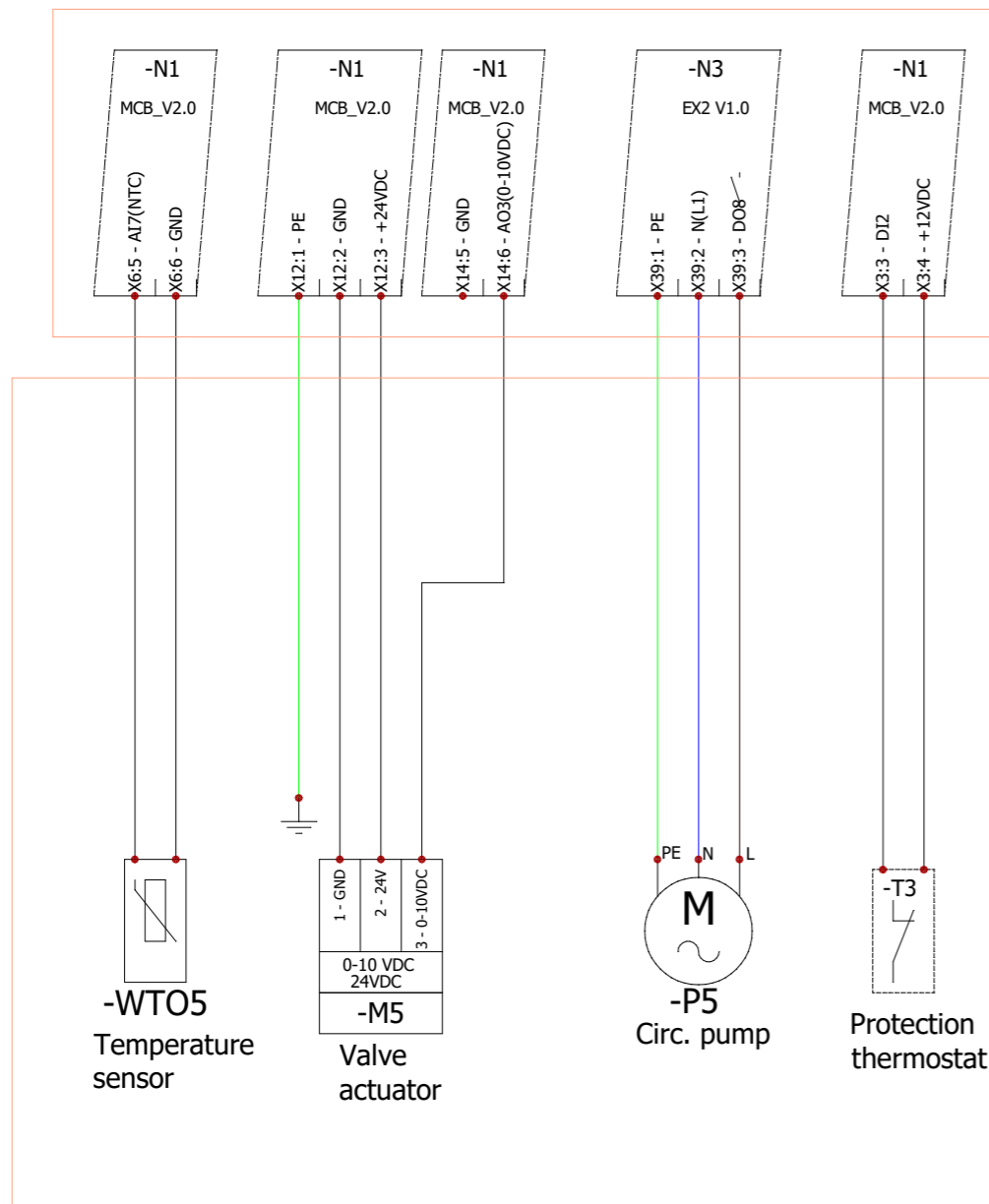
Pav. 4.18.3.3 Išorinio vandens šildytuvo prijungimas
