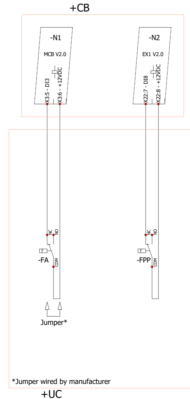
Pav. 4.18.2.2 Priešgaisrinių ir židinių apsaugos jungiklių sujungimas
