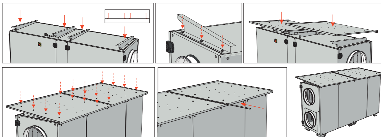
Pav. 4.9.1 Stogo montavimas ant gaminio
