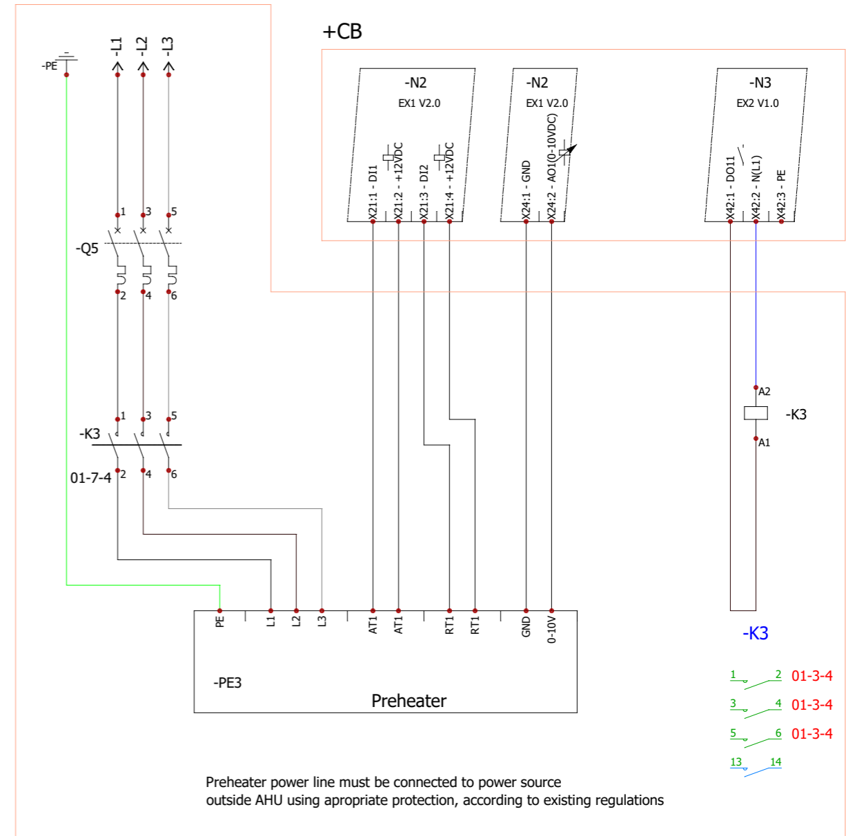
Pav. 4.18.4.1 Išorinio elektrinio pašildytuvo prijungimas
