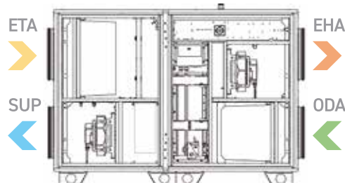
AmberAir Compact S-RH (kairinė versija)
