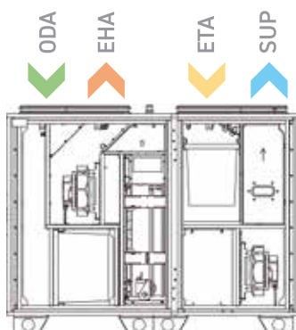
„AmberAir Compact S-RV“ (dešininė versija)
