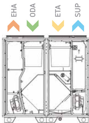
AmberAir Compact S-CXV (dešininė versija)
