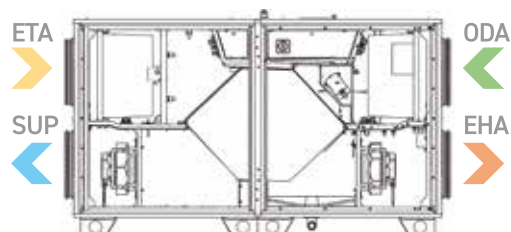
AmberAir Compact S-CXH (kairinė versija)
