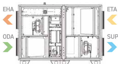
AmberAir Compact S-RH (dešininė versija)
