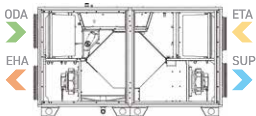
AmberAir Compact S-CXH (dešininė versija)
