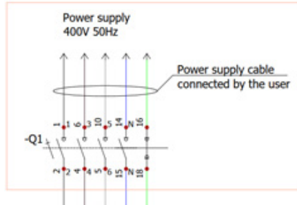
Abbildung 5.9.2. Geräte mit 3N~ 400VAC Stromversorgung
