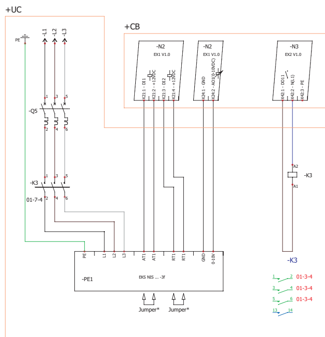
Abbildung 8.9.1. Externes Elektrovorheizregister
