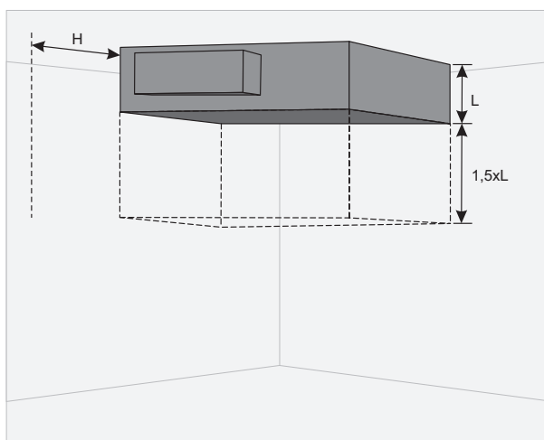
Abbildung 5.6.1. Min. Abstand für Türöffnung - 1,5 \times L ; Min. Abstand für Öffnung des Schaltkastens - H > 400 \text{ mm} .
