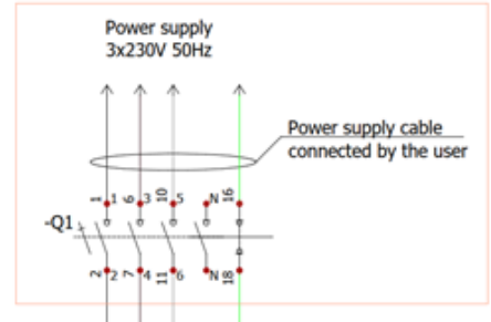
Abbildung 5.9.3. Geräte mit 3~ 230VAC Stromversorgung
