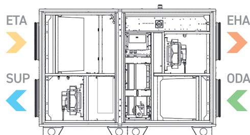
AmberAir Compact S-RH (vasak versioon)
