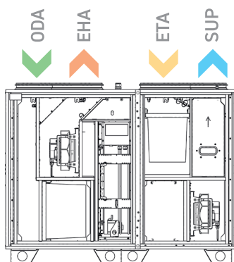
AmberAir Compact S-RV (parem versioon)
