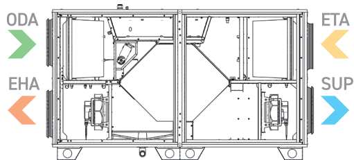
AmberAir Compact S-CXH (parem versioon)
