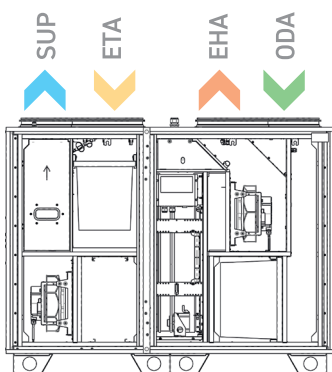
AmberAir Compact S-RV (vasak versioon)
