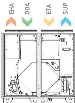
AmberAir Compact S-CXV (parem versioon)
