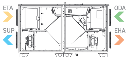
AmberAir Compact S-CXH (vasak versioon)
