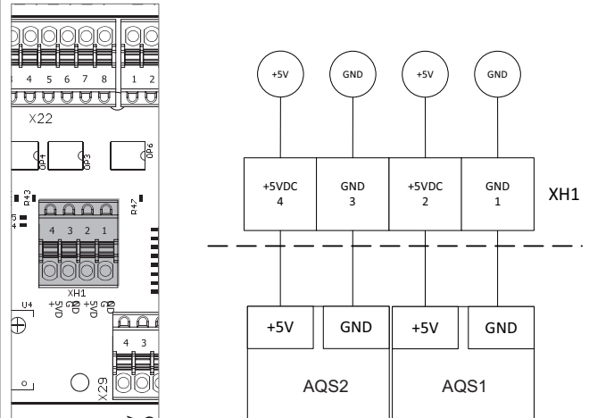
AQS - Captur de qualité de l'air
