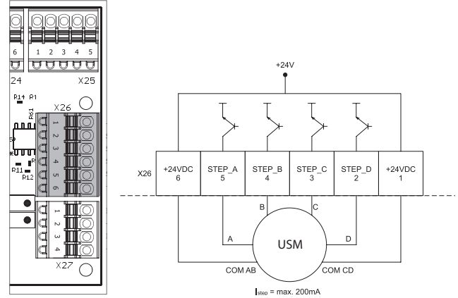
USM - Moteur unipolaire pas à pas
