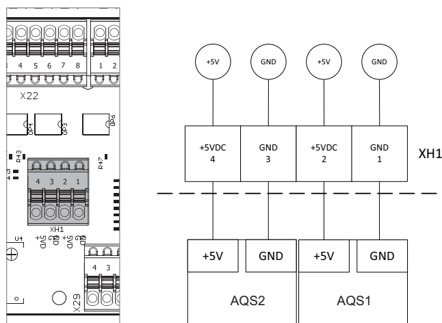
AQS - oro kokybės jutiklis
