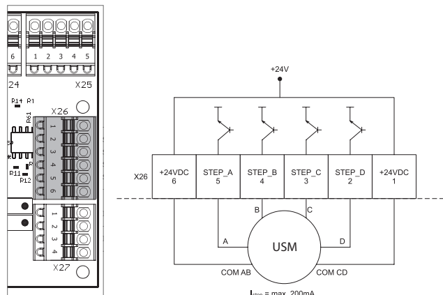
USM - vieno poliariškumo žingsninis variklis
