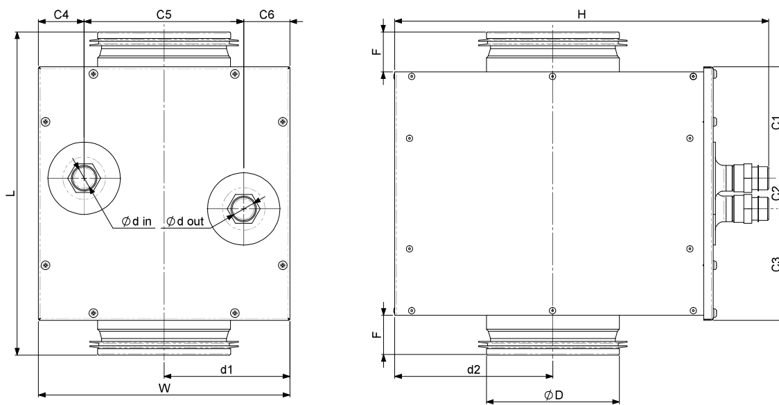
Abb. 10.1 - AVS abmessungen
