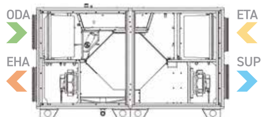
AmberAir Compact S-RH (höger variant)
