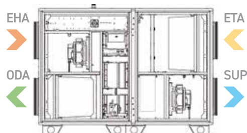
AmberAir Compact S-CXH (höger variant)
