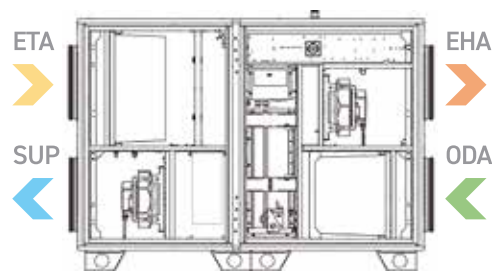
AmberAir Compact S-CXH (vänster variant)
