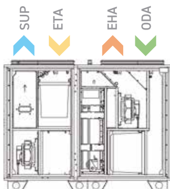
AmberAir Compact S-RV (vänster variant)
