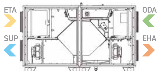
AmberAir Compact S-RH (vänster variant)
