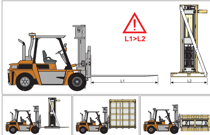
Figuur 5.2.2. Hijsen d.m.v. vorkheflift AmberAir Compact RIS 1900-2500 P EKO 3.0
