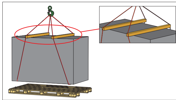
Figuur 5.2.3. Hijsen AmberAir Compact RIS 1200 P EKO 3.0
