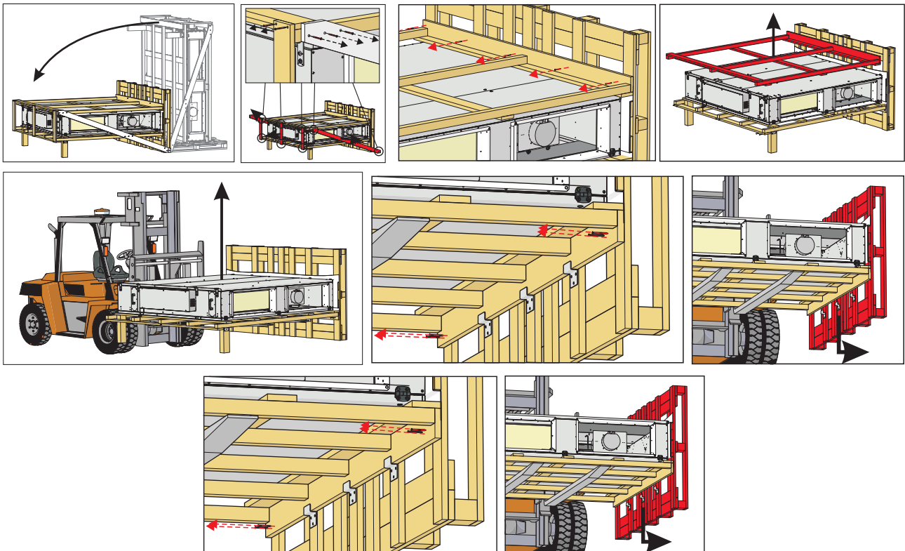
Figuur 5.3.2. Uitpakken AmberAir Compact RIS 1900-2500 P EKO 3.0
