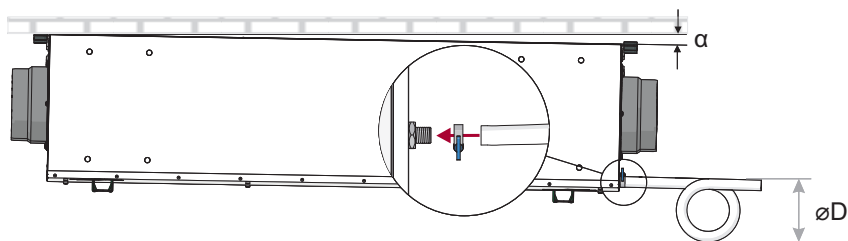
Figuur 5.5.2.2. Installatie condensafvoersysteem ( \varnothing D=150 mm)
