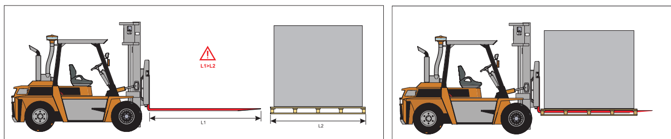
Figuur 5.2.1. Hijsen d.m.v. vorkheflift AmberAir Compact RIS 1200 P EKO 3.0
