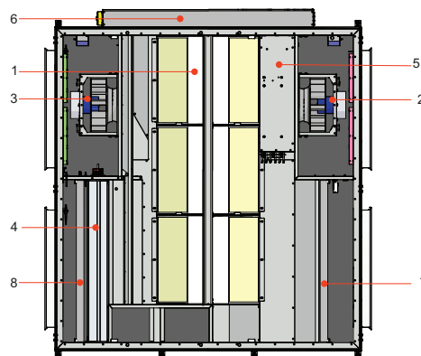
Figuur 4.2. AmberAir Compact RIS 1900-2500 P EKO 3.0
