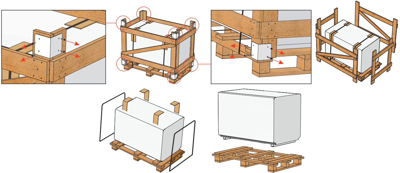
Figuur 5.3.1. Uitpakken AmberAir Compact RIS 1200 P EKO 3.0
