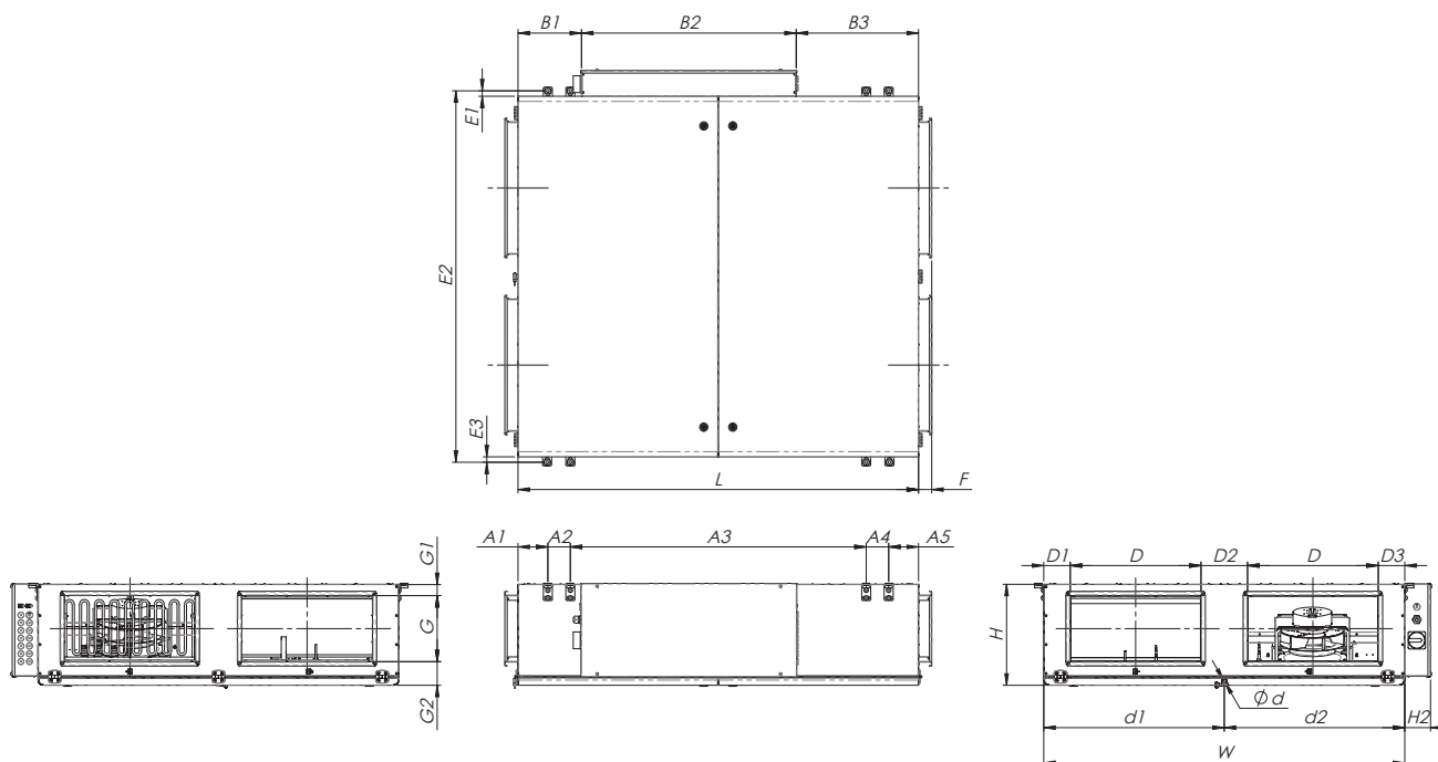
Figuur 4.2.1. AmberAir Compact RIS 1200 P EKO 3.0 afmetingen
