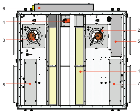
Figuur 4.1. AmberAir Compact RIS 1200 P EKO 3.0
