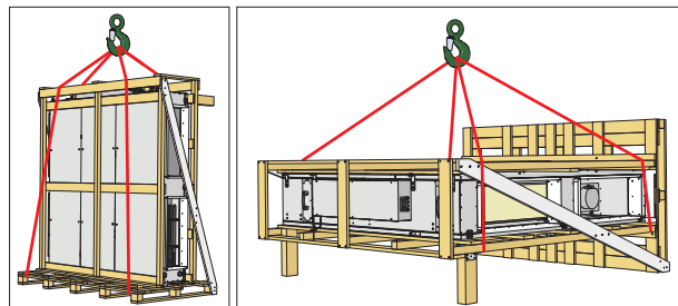
Figuur 5.2.4. Hijsen AmberAir Compact RIS 1900-2500 P EKO 3.0
