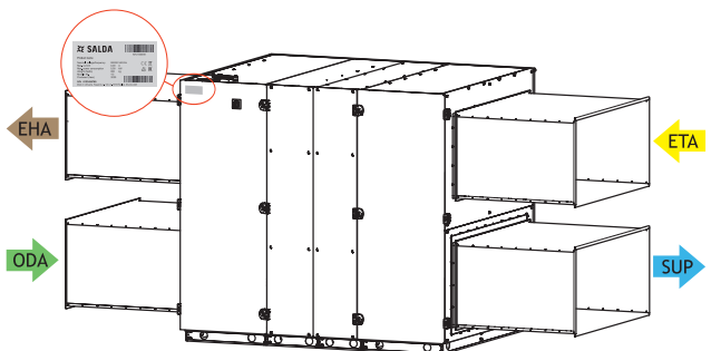
Fig. 3.3.8 Umieszczenie etykiety technicznej i oznaczenie króćców powietrza AmberAir Compact-S-R-7000-9000-H (prawa strona)
