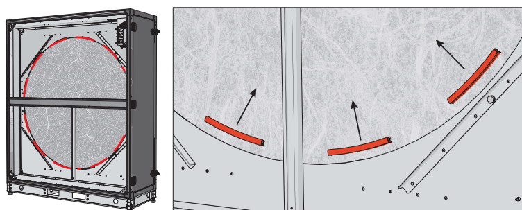
Fig. 4.5.3 Usuwanie gumowych taśm do transportu (tylko dla AmberAir Compact S-R-7000-9000-H)
