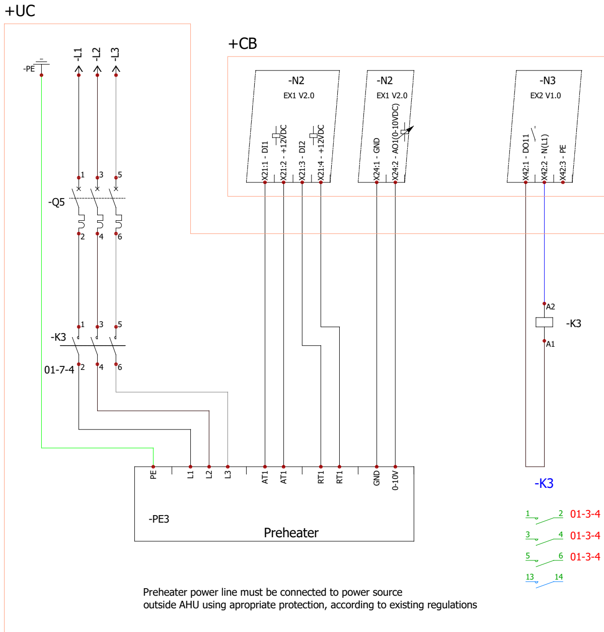
Fig. 4.19.4.1 Podłączenie zewnętrznej elektrycznej nagrzewnicy wstępnej
