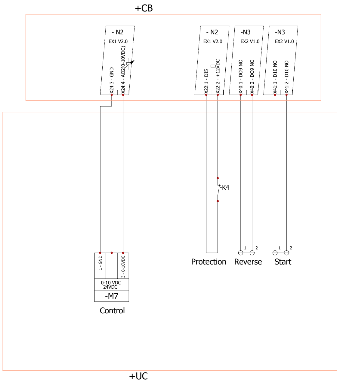
Fig. 4.19.3.1 Podłączenie zewnętrznej chłodnicy DX
