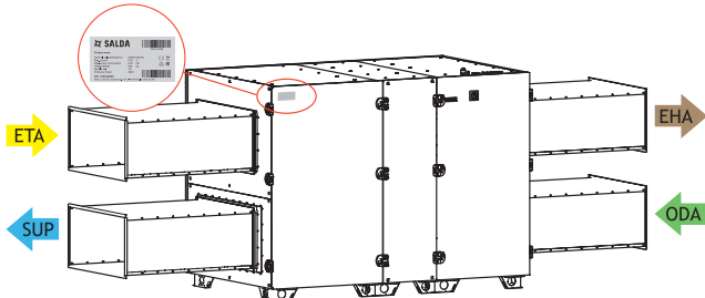
Fig. 3.3.5 Umieszczenie etykiety technicznej i oznaczenie króćców powietrza AmberAir Compact-S-R-3000-4000-5000-H (lewa strona)
