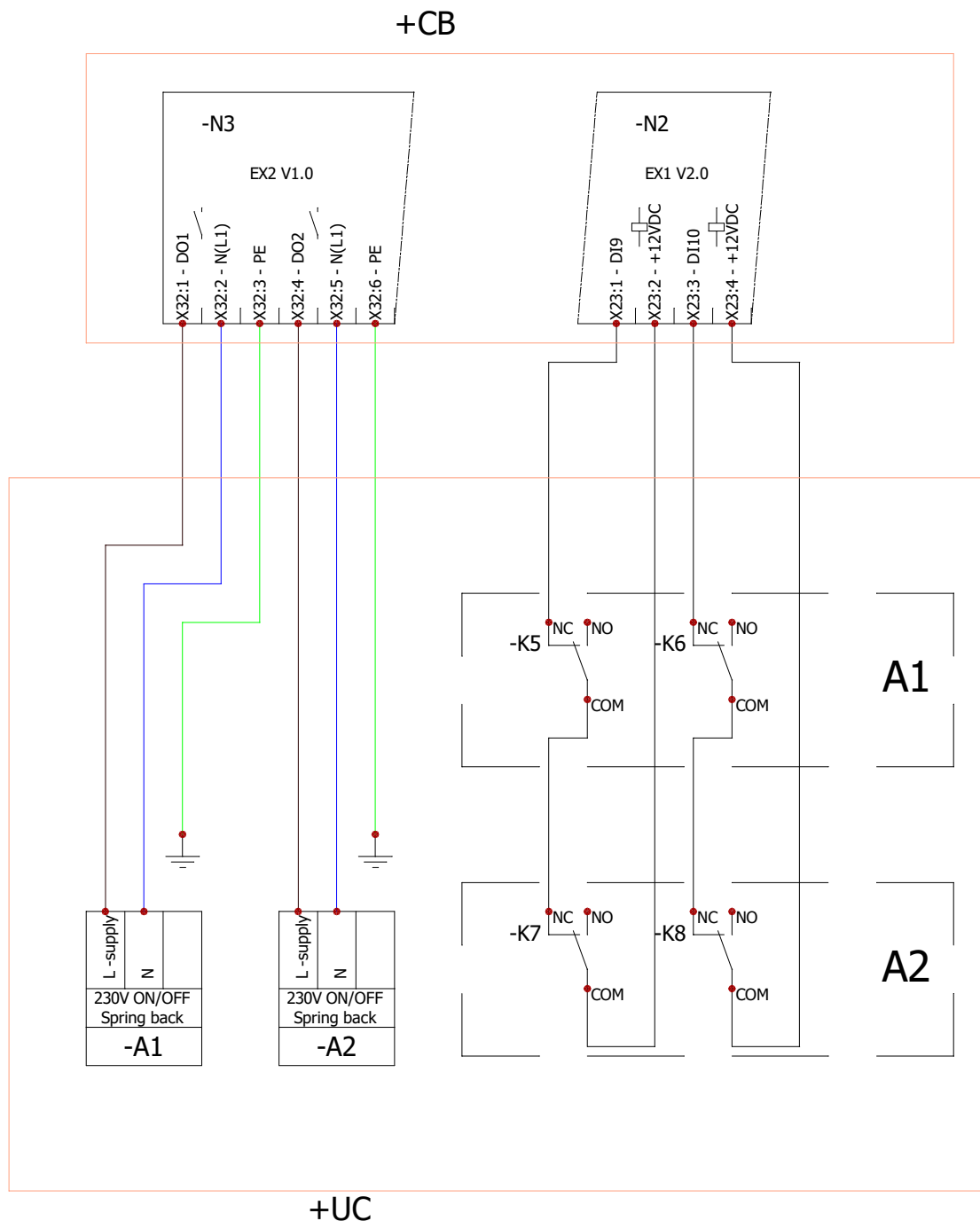
Fig. 4.19.2.1 Podłączenie klap przeciwpożarowych i czujników położenia
