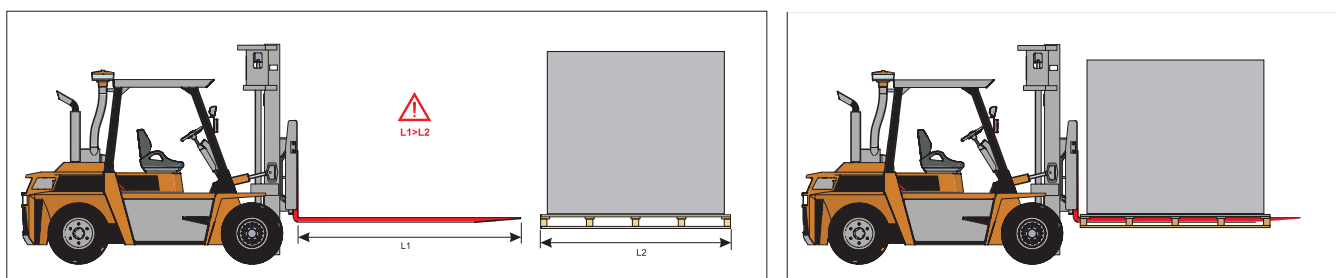
Fig. 4.3.1 AmberAir Compact S-R-1000-9000 podnoszenie wózkiem widłowym
