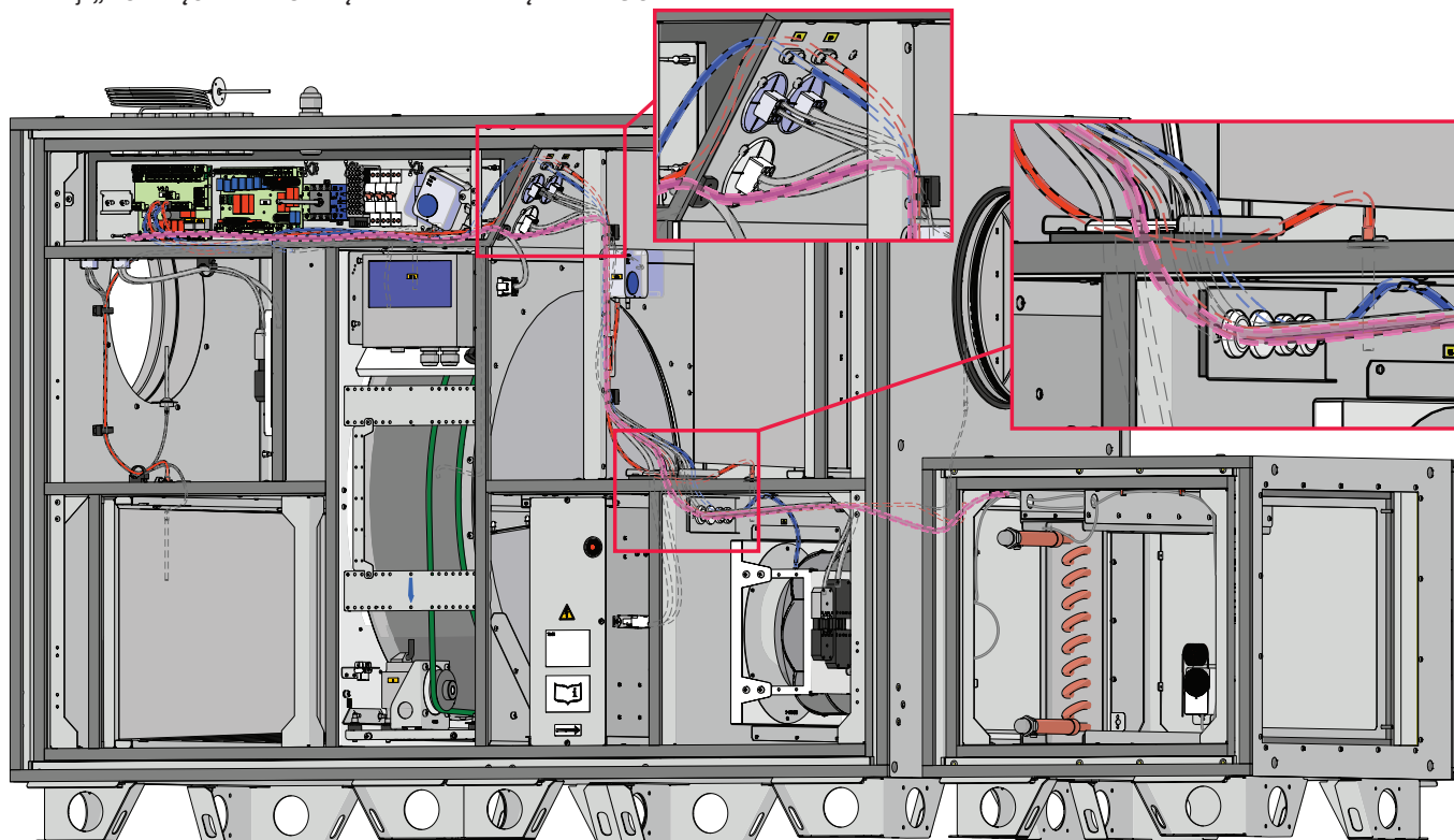
Fig. 4.13.1 Zewnętrzny grzejnik/chłodnica (Comfort Box) prowadzenie kabli dla AmberAir Compact S-R-1000-2000-H
