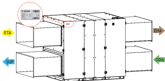
Fig. 3.3.7 Umieszczenie etykiety technicznej i oznaczenie króćców powietrza AmberAir Compact-S-R-7000-9000-H (lewa strona)
