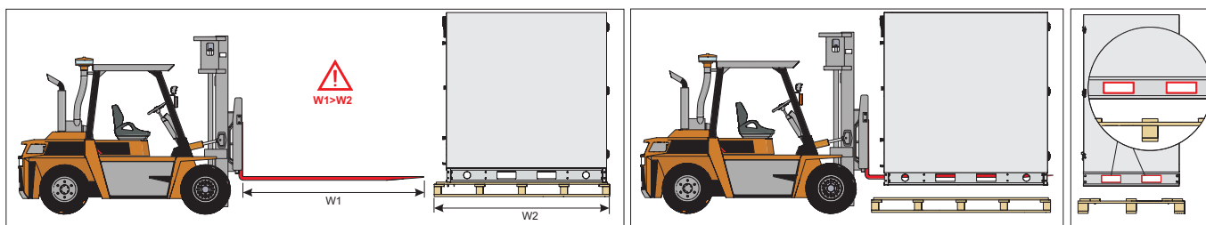
Fig. 4.3.2 AmberAir Compact S-R-7000-9000 podnoszenie wózkiem widłowym
