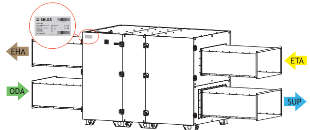
Fig. 3.3.6 Umieszczenie etykiety technicznej i oznaczenie króćców powietrza AmberAir Compact-S-R-3000-4000-5000-H (prawa strona)
