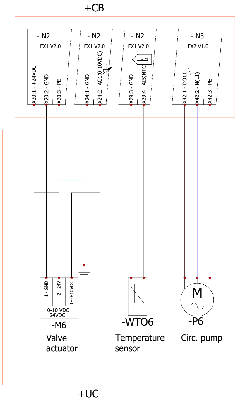
Fig. 4.19.4.2 Podłączenie zewnętrznej wstępnej nagrzewnicy wody
