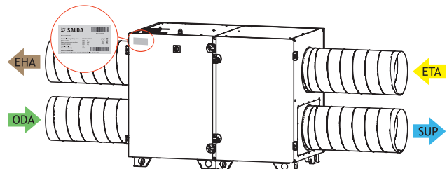
Fig. 3.3.4 Umieszczenie etykiety technicznej i oznaczenie króćców powietrza AmberAir Compact-S-R-1000-1500-2000-H (prawa strona)
