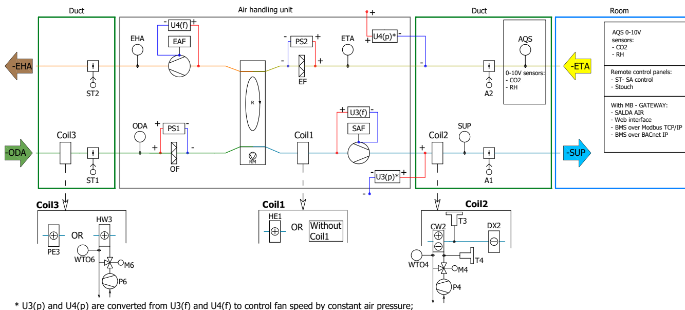
Fig. 8.6.1 Centrale poziome prawostronne ze zintegrowaną nagrzewnicą elektryczną lub bez zintegrowanej nagrzewnicy/chłodziцы
