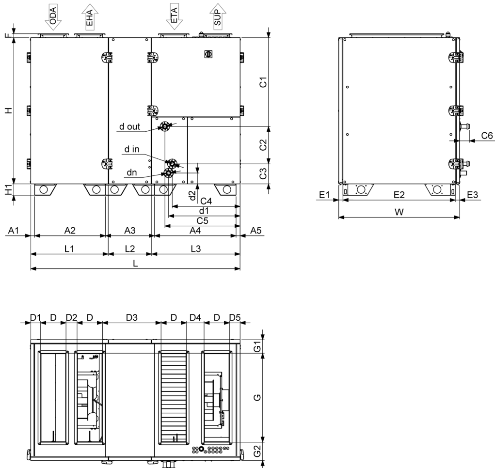
Fig. 8.1.10 AmberAir Compact-S-R-2000-V-CO-R-C1 / AmberAir Compact-S-R-3000-V-CO-R-C1 / AmberAir Compact-S-R-4000-V-CO-R-C1 / AmberAir Compact-S-R-5000-V-CO-R-C1 dimensioner
