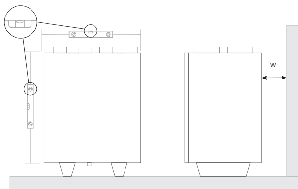
Fig. 4.7.1 Horisontell positioner vid golvmontering (W=400 mm)
