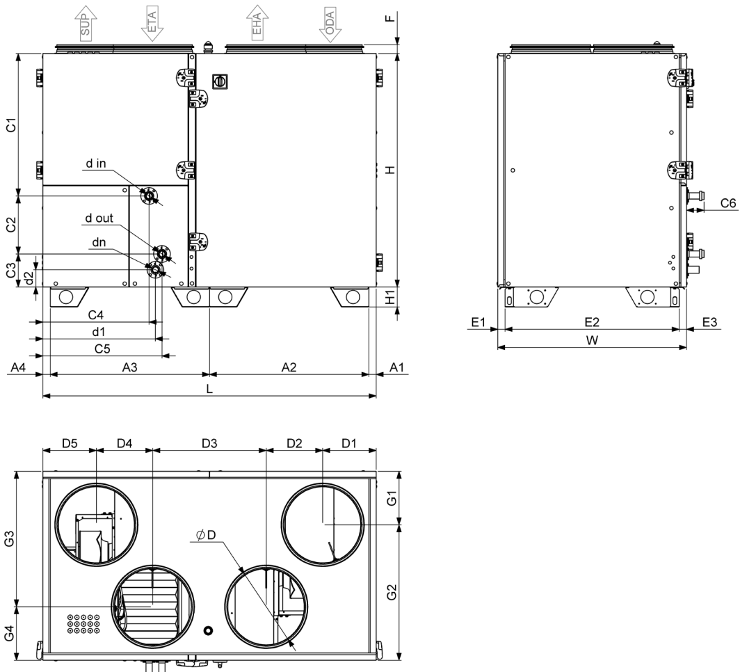
Fig. 8.1.3 AmberAir Compact S-R-1000-V-CO-L-C1 / AmberAir Compact S-R-1500-V-CO-L-C1 dimensioner
