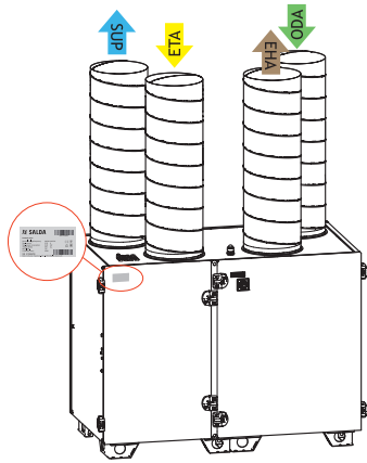
Fig. 3.3.3 Placering av typskylt och anslutning av luftkanaler AmberAir Compact-S-R-1000-1500-V (vänster version)
