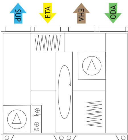
Fig. 3.4.1 AmberAir Compact S-R V (vänster version)
