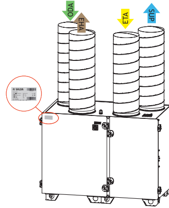
Fig. 3.3.4 Placering av typskylt och anslutning av luftkanaler AmberAir Compact-S-R-1000-1500-V (höger version)
