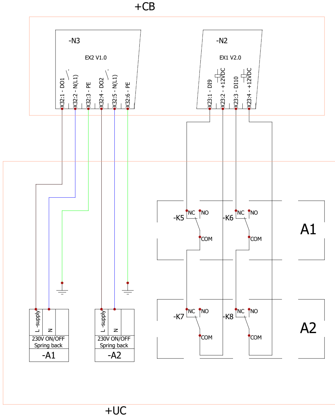
Fig. 4.15.2.1 Brandspjäll och anslutning av lägesbrytare
