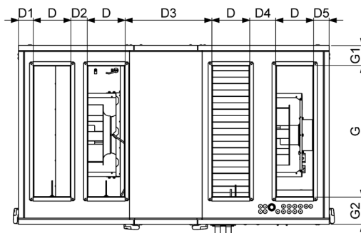
Fig. 8.1.12 AmberAir Compact-S-R-2000-V-DX-R-C1 / AmberAir Compact-S-R-3000-V-DX-R-C1 / AmberAir Compact-S-R-4000-V-DX-R-C1 / AmberAir Compact-S-R-5000-V-DX-R-C1 dimensioner
