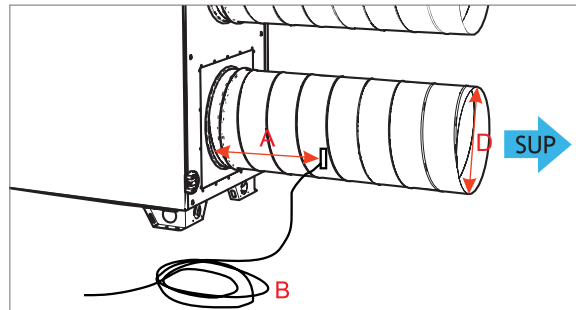
Fig. 4.10.1 A – 3 x D; B – 6 m (A – min. avstånd; B – kabellängd; D – kanaldiameter).
