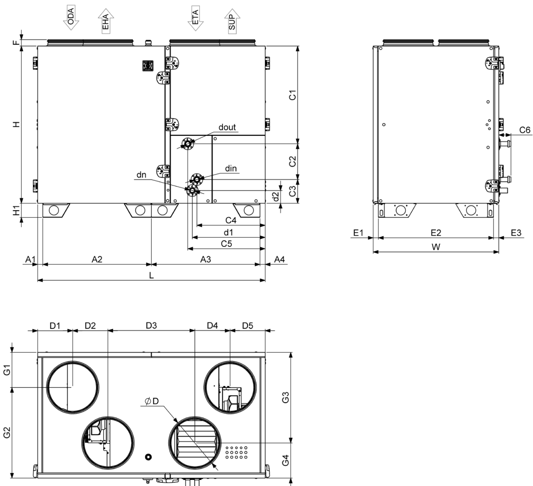
Fig. 8.1.4 AmberAir Compact S-R-1000-V-CO-R-C1 / AmberAir Compact S-R-1500-V-CO-R-C1 dimensioner
