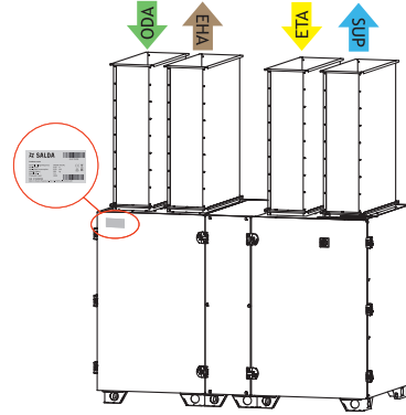
Fig. 3.3.6 Placering av typskylt och anslutning av luftkanaler AmberAir Compact-S-R-2000-3000-4000-5000-V (höger version)
