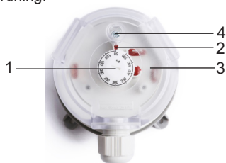
1 - Tryckinställningsratt; 2 - Markering; 3 - Hölje; 4 - Fästskruvar.
