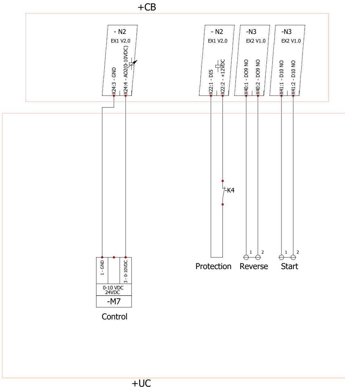
Fig. 4.15.3.1 Anslutning till extern DX-kylare
