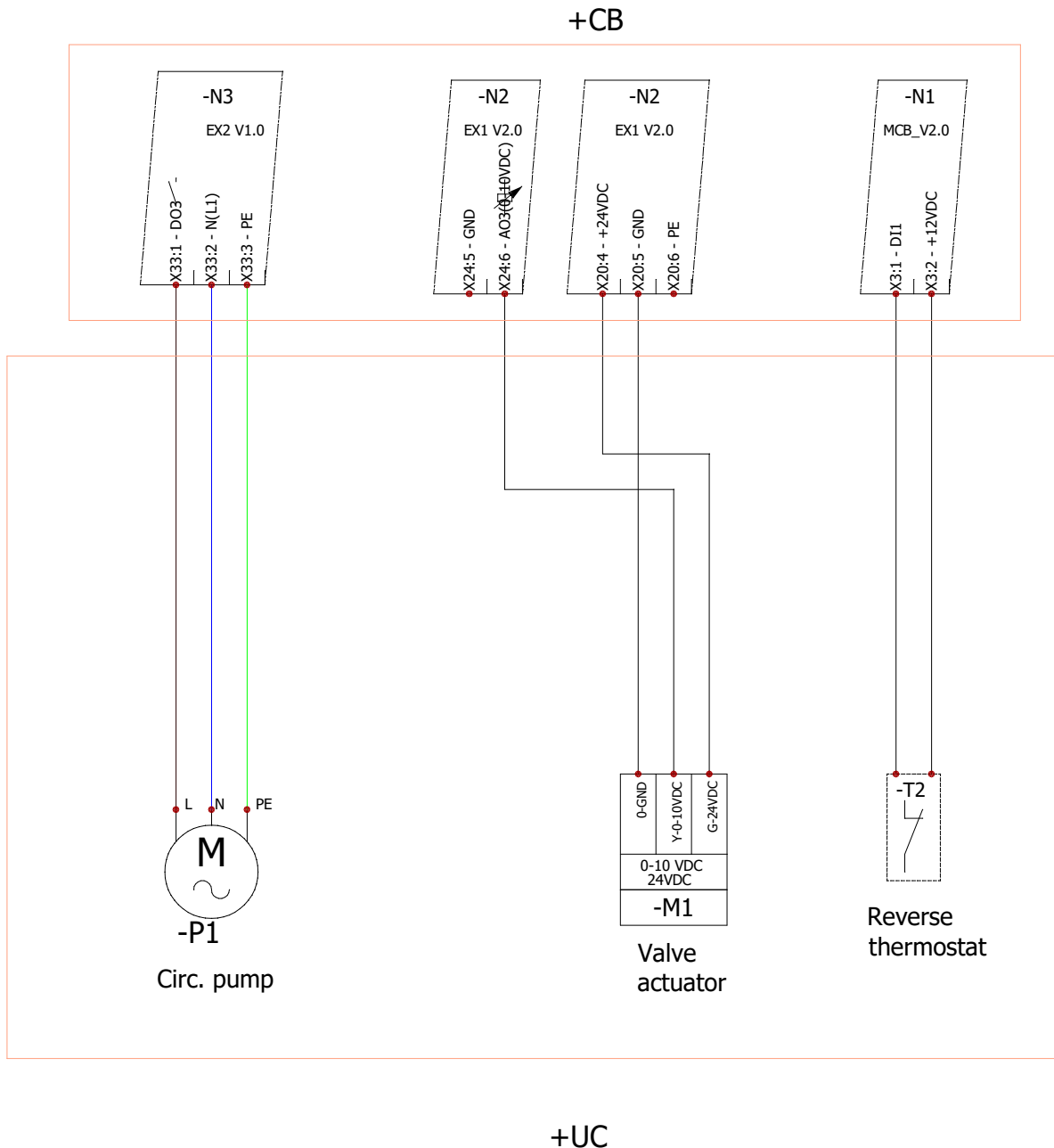
Fig. 4.15.6.1 Anslutning av tillbehör för intern kombinerad värme-/kylarslinga
