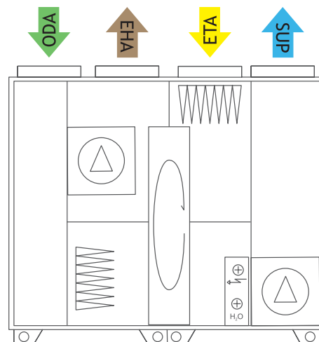
Fig. 3.4.2 AmberAir Compact S-R V (höger version)
