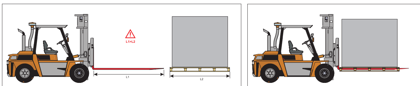
Fig. 4.3.1 Lyft av AmberAir Compact med gaffeltruck
