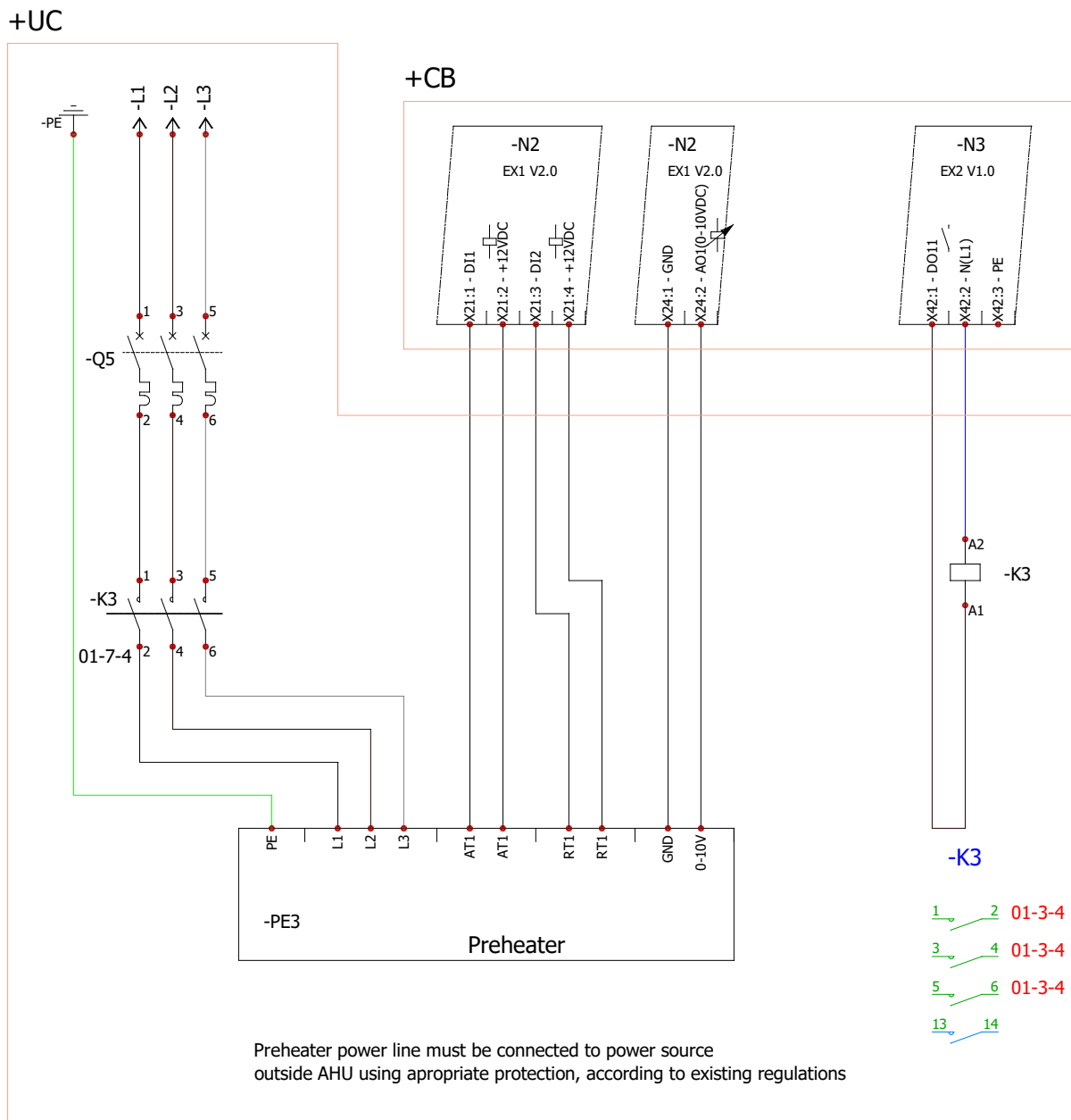
Fig. 4.15.4.1 Anslutning till extern elektrisk förvärmare
