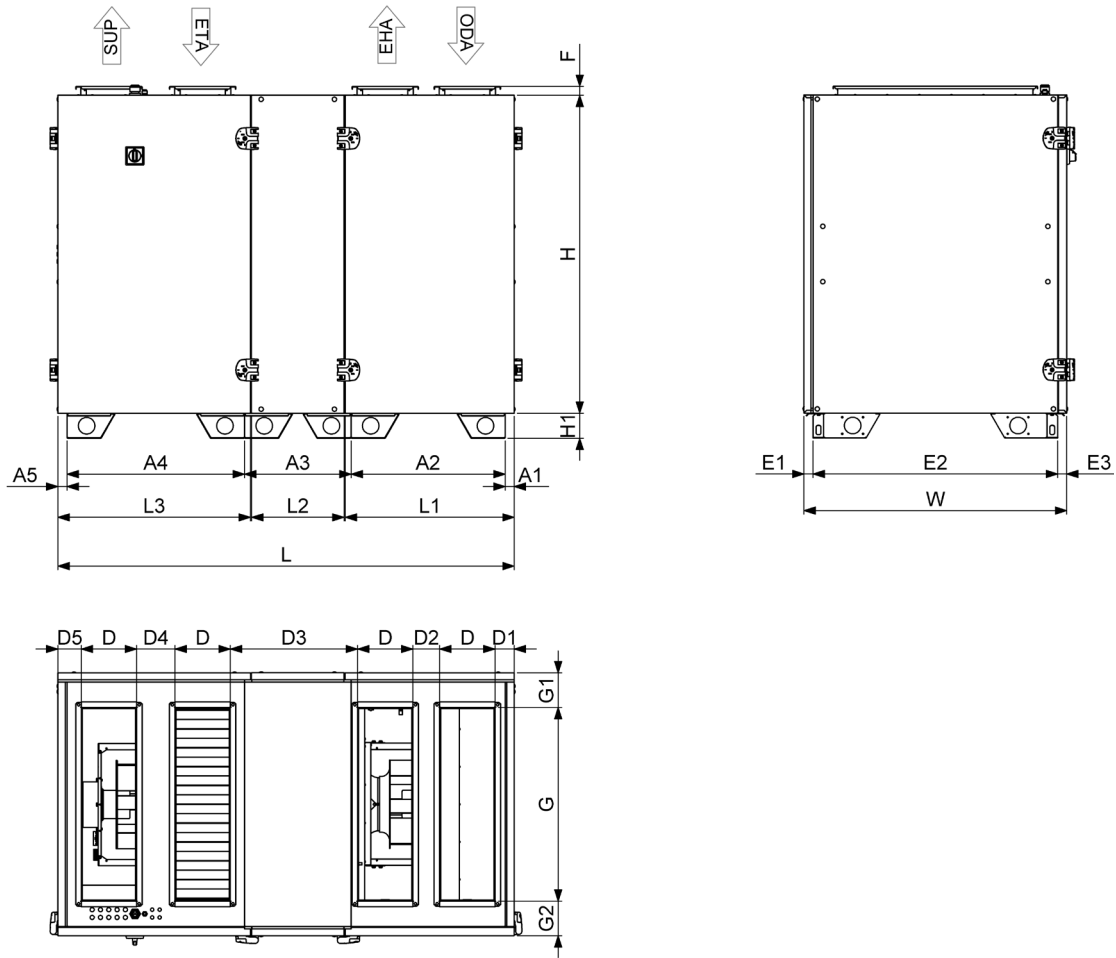
Fig. 8.1.7 AmberAir Compact-S-R-2000-V-E-L-C1 / AmberAir Compact-S-R-3000-V-E-L-C1 / AmberAir Compact-S-R-4000-V-E-L-C1 / AmberAir Compact-S-R-5000-V-E-L-C1 dimensioner
