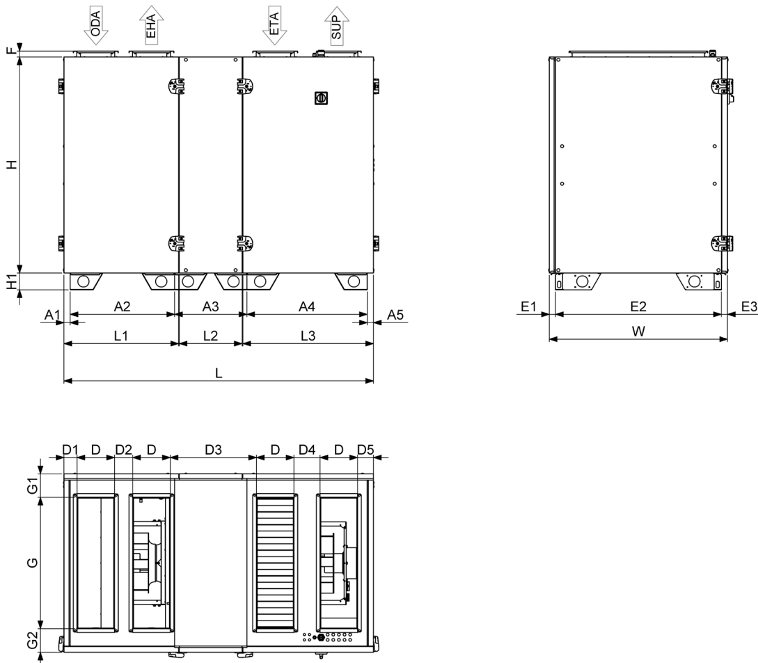
Fig. 8.1.8 AmberAir Compact-S-R-2000-V-E-R-C1 / AmberAir Compact-S-R-3000-V-E-R-C1 / AmberAir Compact-S-R-4000-V-E-R-C1 / AmberAir Compact-S-R-5000-V-E-R-C1 dimensioner
