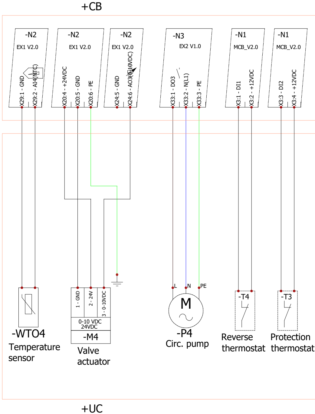
Fig. 4.15.3.2 Anslutning till extern kombinerad värme-/kylarslinga
