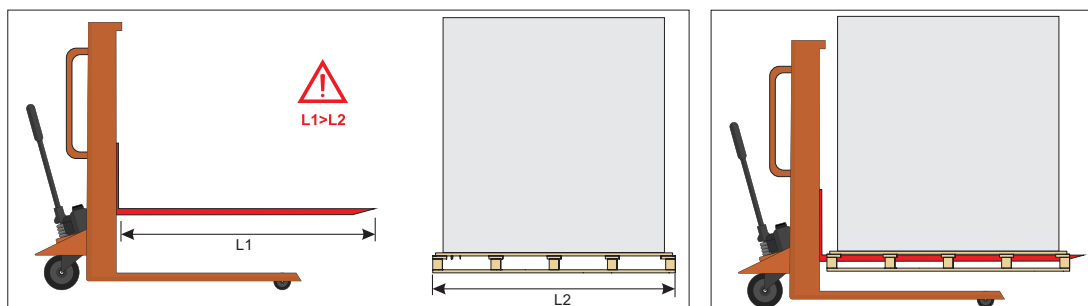
Fig. 4.3.2 Lyft av AmberAir Compact med pallyftare
