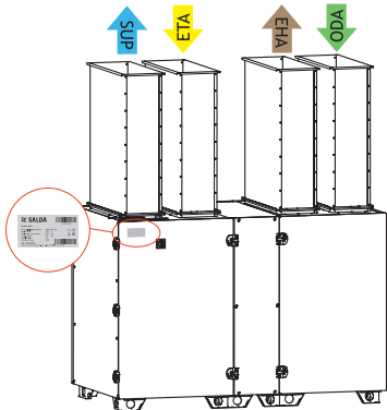
Fig. 3.3.5 Placering av typskylt och anslutning av luftkanaler AmberAir Compact-S-R-2000-3000-4000-5000-V (vänster version)
