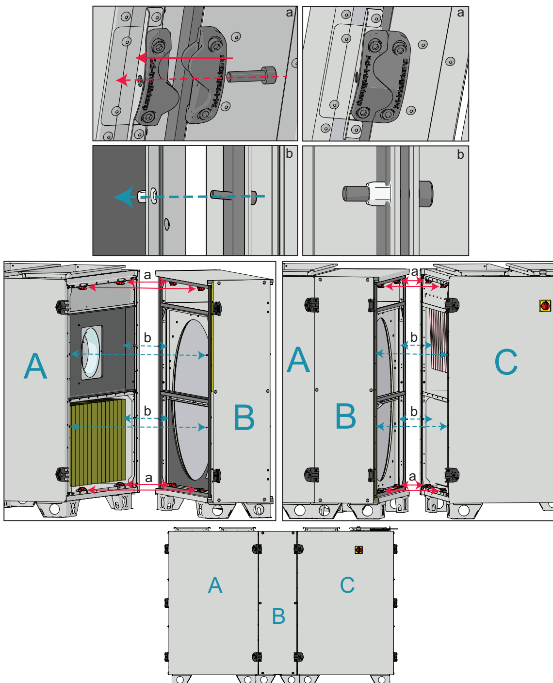
Fig. 4.8.1.1 AmberAir Compact S-R-V – anslutning av sektioner
