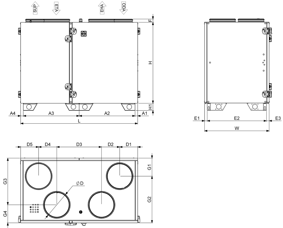
Fig. 8.1.1 AmberAir Compact S-R-1000-V-E-L-C1 / AmberAir Compact S-R-1500-V-E-L-C1 dimensioner
