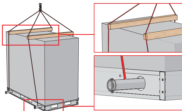
Fig. 4.3.3 Lyfta AmberAir Compact med lyftselar
