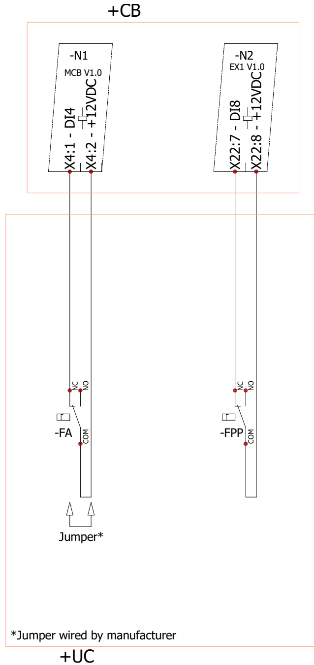
Fig. 4.15.2.2 Brand- och eldstadssäkerhet – anslutning av säkerhetsbrytare
