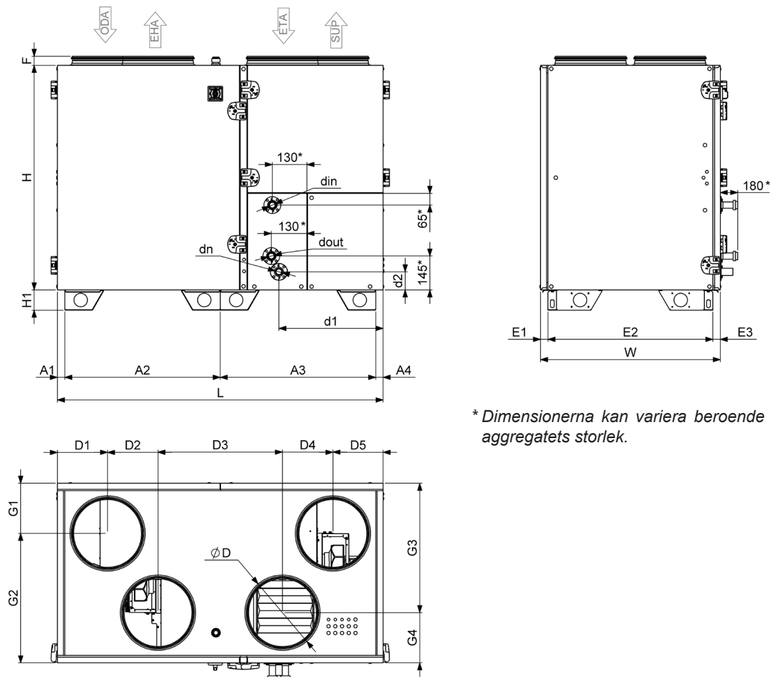
Fig. 8.1.6 AmberAir Compact S-R-1000-V-DX-R-C1 / AmberAir Compact S-R-1500-V-DX-R-C1 dimensioner
