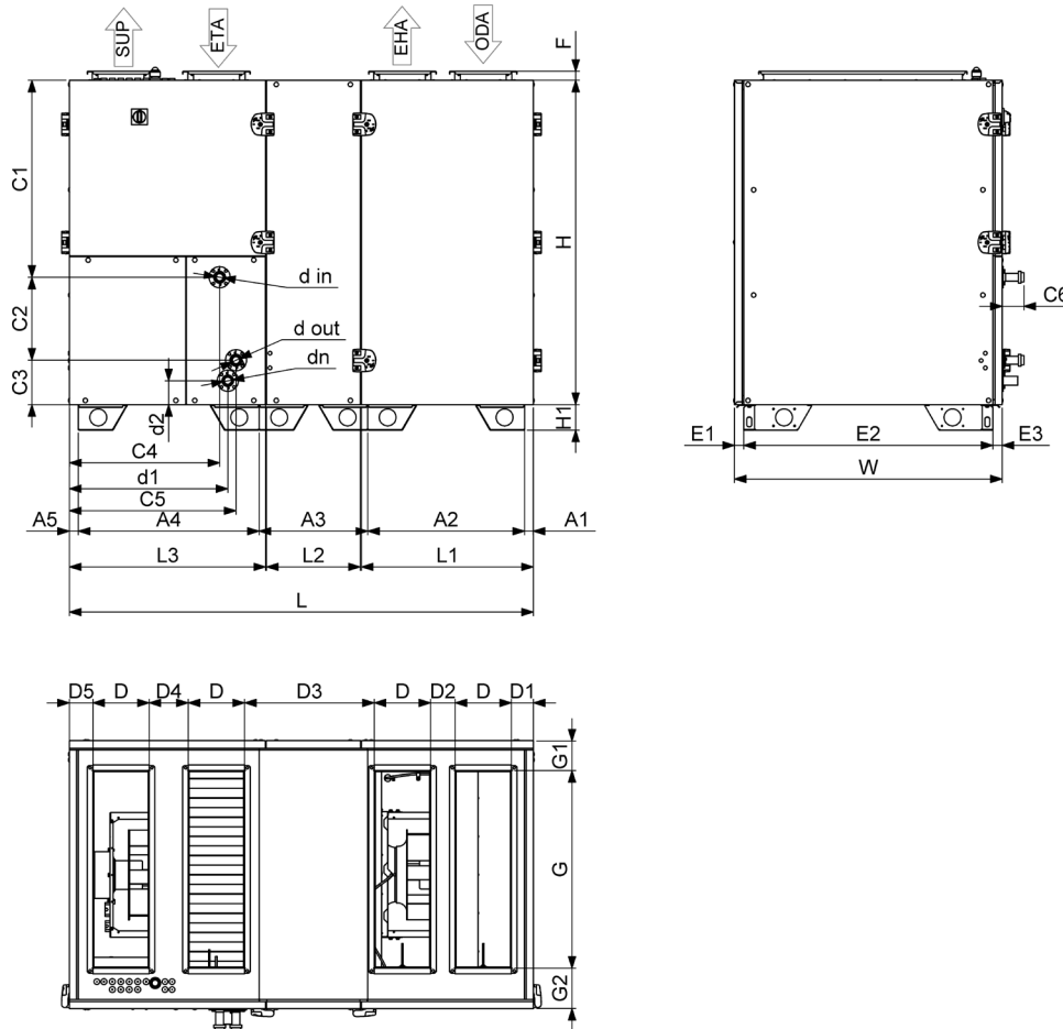
Fig. 8.1.9 AmberAir Compact-S-R-2000-V-CO-L-C1 / AmberAir Compact-S-R-3000-V-CO-L-C1 / AmberAir Compact-S-R-4000-V-CO-L-C1 / AmberAir Compact-S-R-5000-V-CO-L-C1 dimensioner
